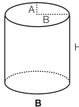
Elliptical Tanks area = 2 · π · (A · B + √((A 2 + B 2 ) / 2) · H) V = π · A · B · H
