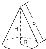
Cone A = π · R · (S + R) V = (π / 180) · R 2 · H
